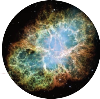
• nebulosa del cranc
