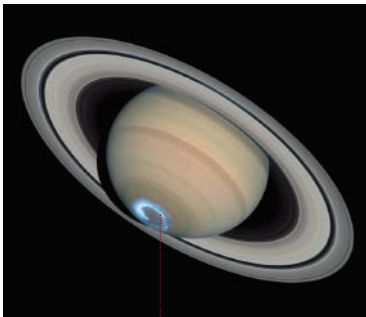
• Saturn amb aurora
