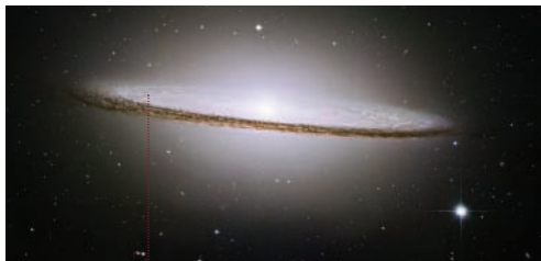
galàxia del barret M/104
