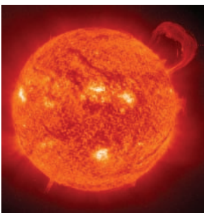
• Sol amb protuberància
