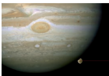
Júpiter amb lluna
